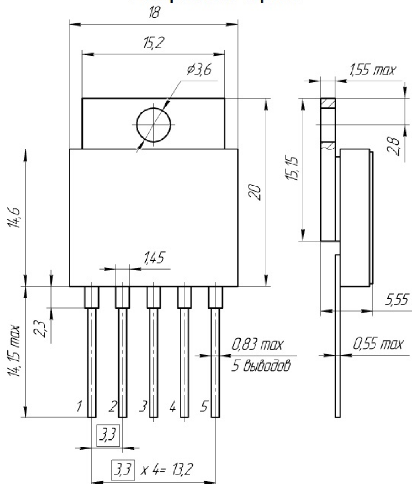
Габаритный чертеж
