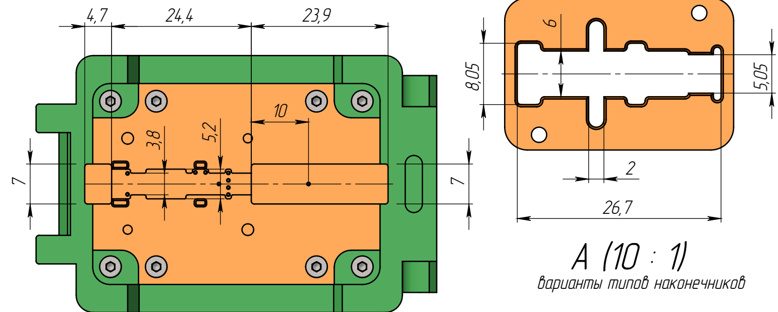
Ограничитель для платы
