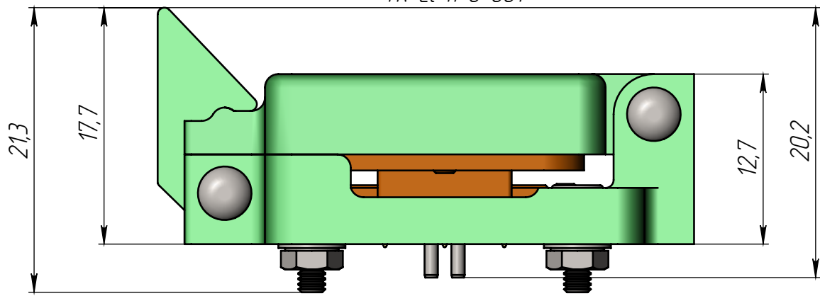
Внешний вид и габаритные размеры КУ TK-cl-h-6-001
