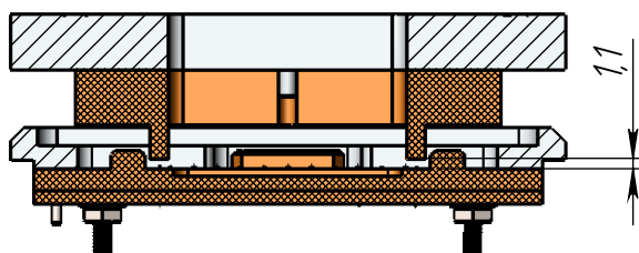
Вариант прижима "2"
