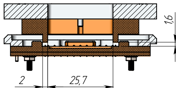
Вариант прижима "1"
