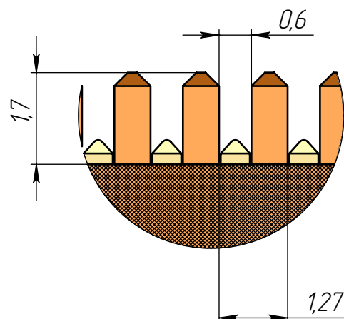
Гребенка (увеличено)
