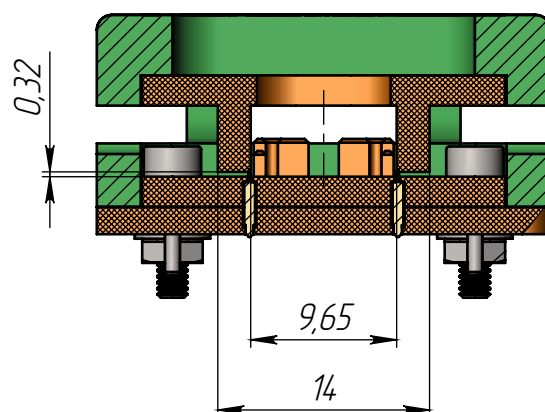
Гребенка (увеличено)
