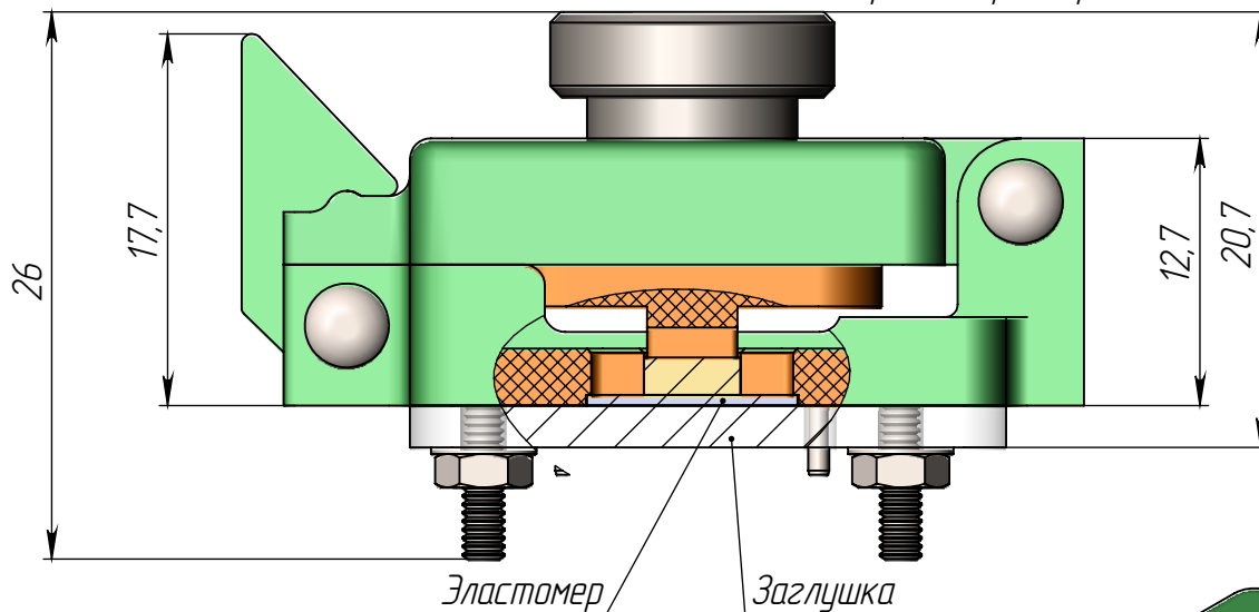
Внешний вид и габаритные размеры КУ
