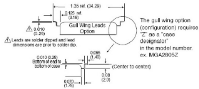
CASE D1 GULL-WING PADS
