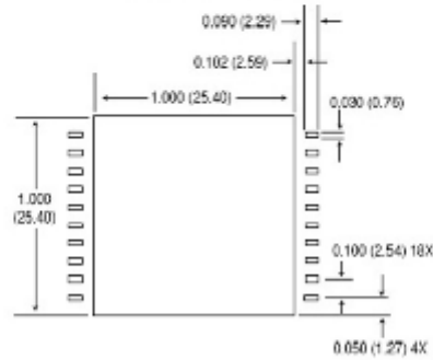
CASE D1 GULL-WING PADS
