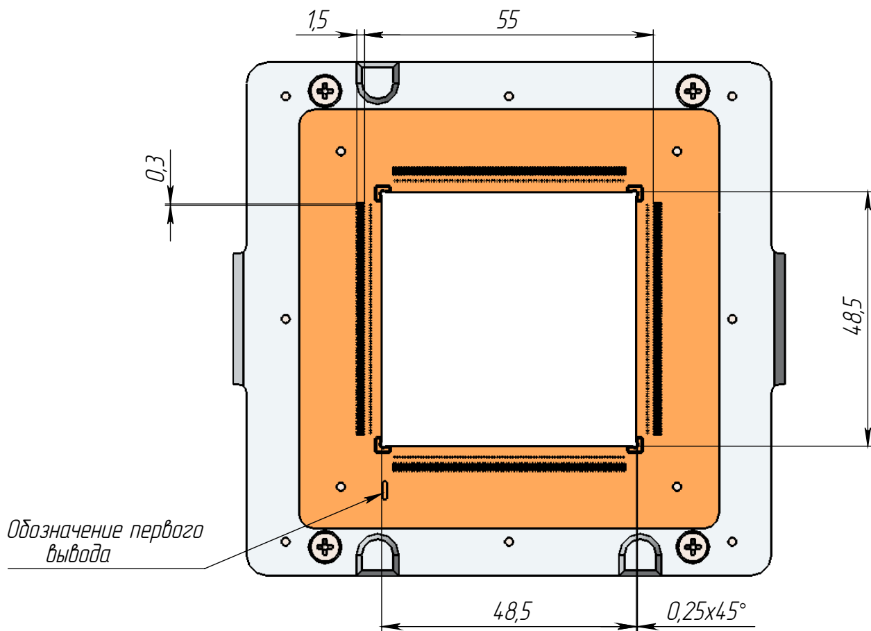
Вид без крышки
