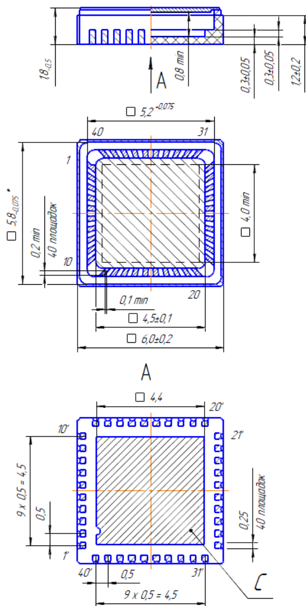
Габаритный чертеж корпуса QLCC 40/40-1
