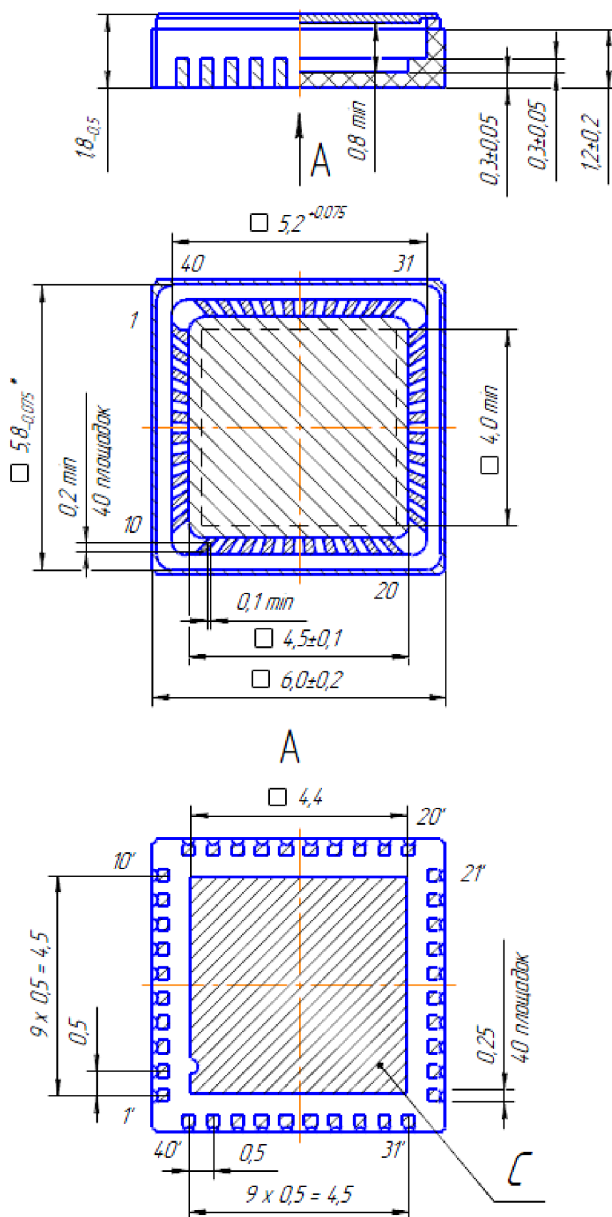
Габаритный чертеж корпуса QLCC 40/40-1
