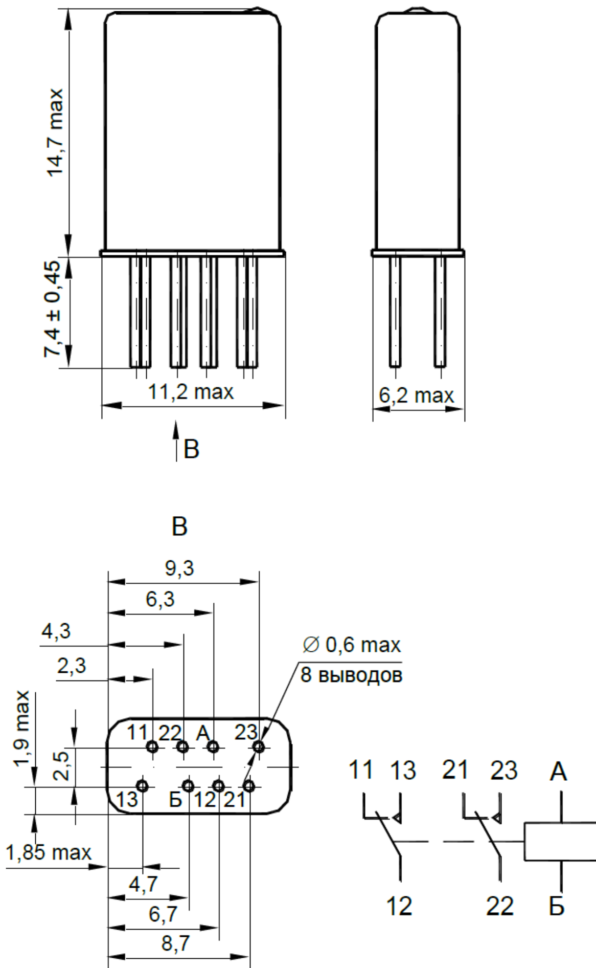
Рис. 4. Внешний вид и габариты ЭРИ (предоставляется заказчиком)
