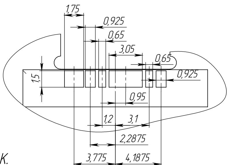
B (5 : 1)
