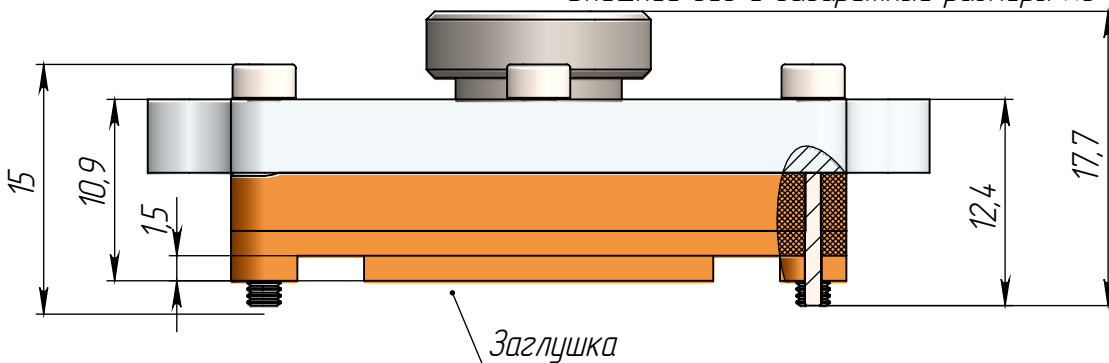
Внешний вид и габаритные размеры КУ
