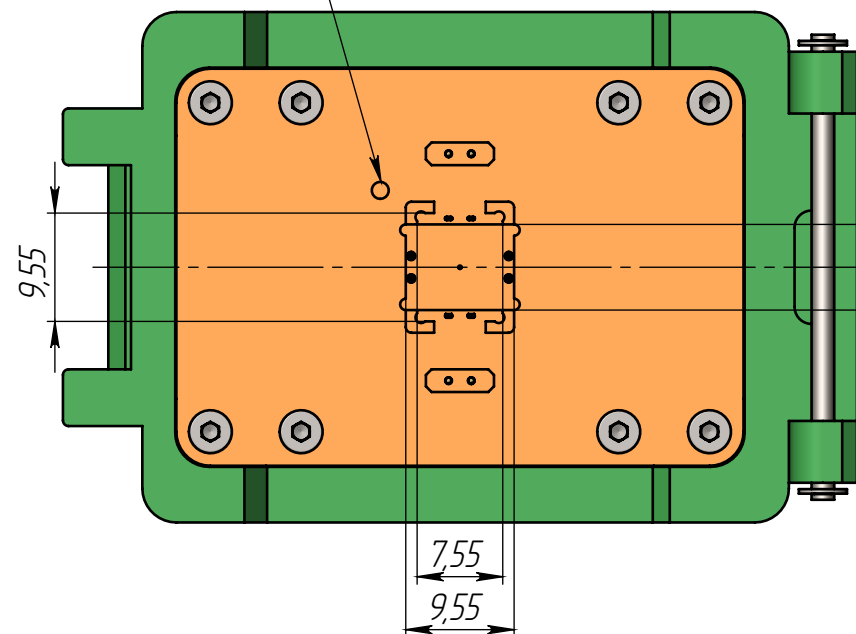
Обозначение первого вывода
