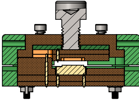
Свободное положение
