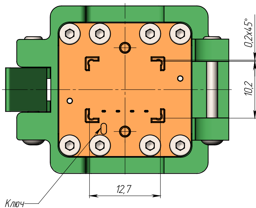
Вид без крышки
