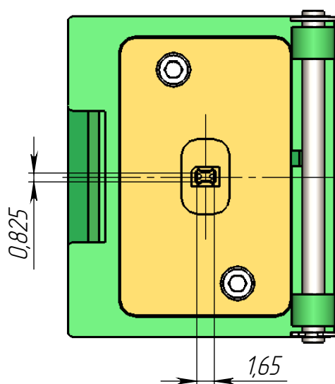
Вид без крышки
