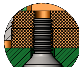
Крепление КУ к печатной плате
