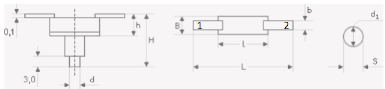
Резисторы P1-3-10 и P1-3-25
