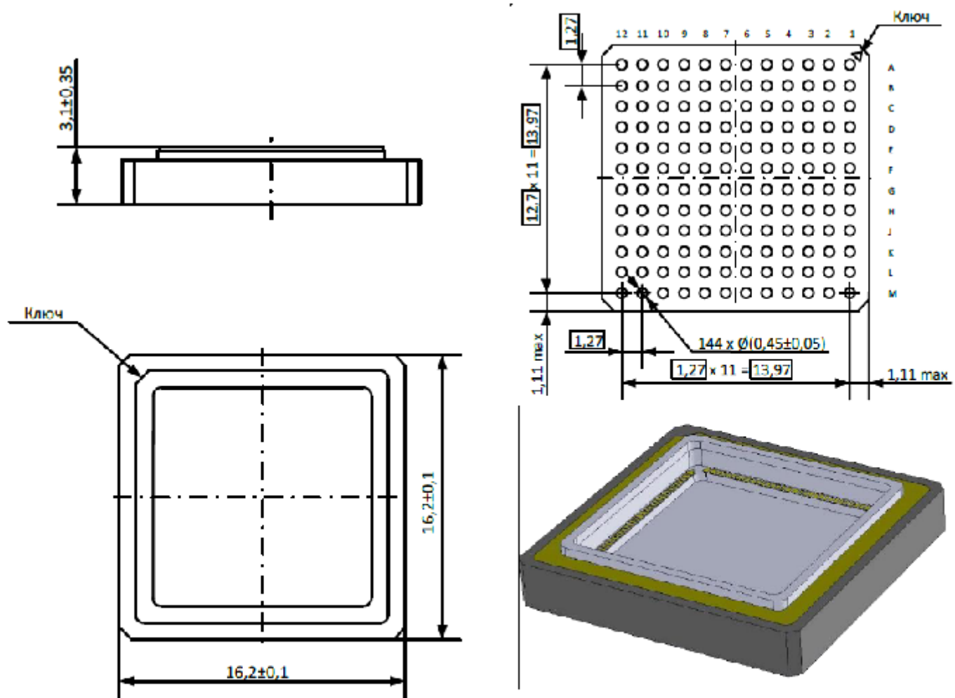
Габаритный чертеж
