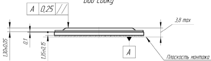
Вид сбоку
