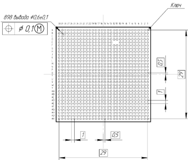
Вид снизу
